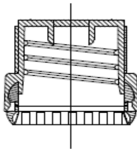
装配图
